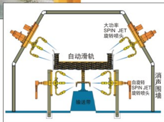
SPIN JET 自动清洗旋转喷射头，可节省人工
